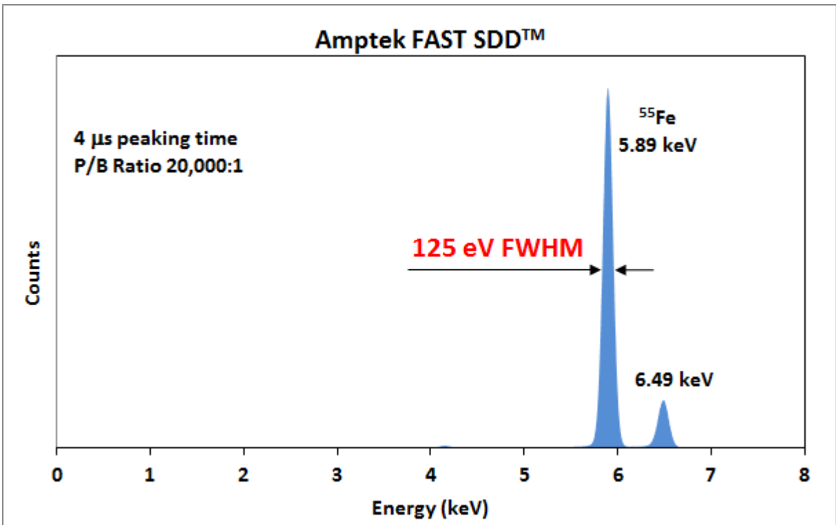
图 4，使用快速 SDD™ 测试 Fe 55 光谱
