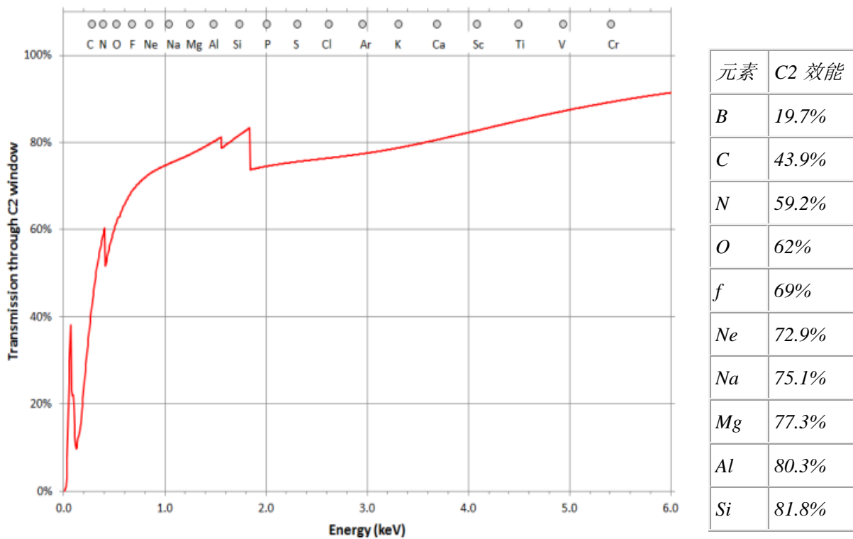
图 2, C2 窗口传输效能图
