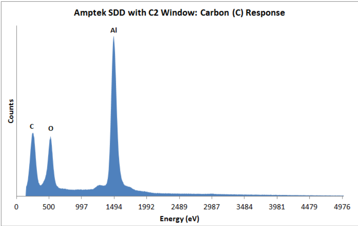
图 3，在真空环境下使用快速 SDD™配 C2 窗口，碳(C)元素光谱图
