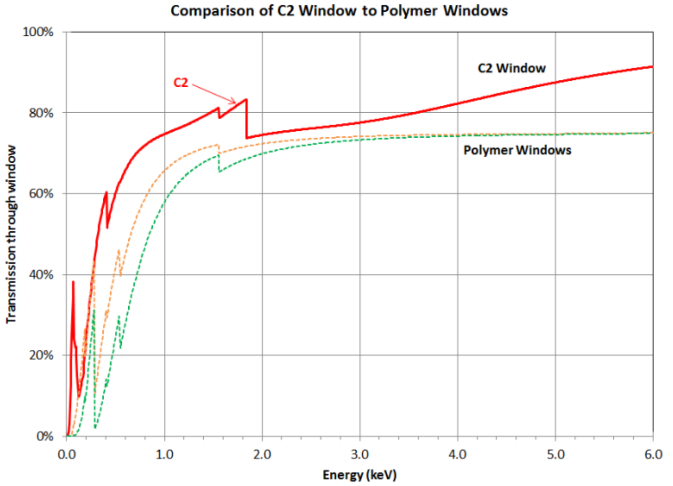
图 4，Amptek 低能量 C2 系列窗口对比聚合物窗口效能图
